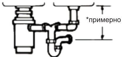
ЦЕНТРАЛЬНЫЙ СЛИВ
